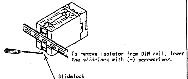
Fig.4 DIN Rail Mounting
